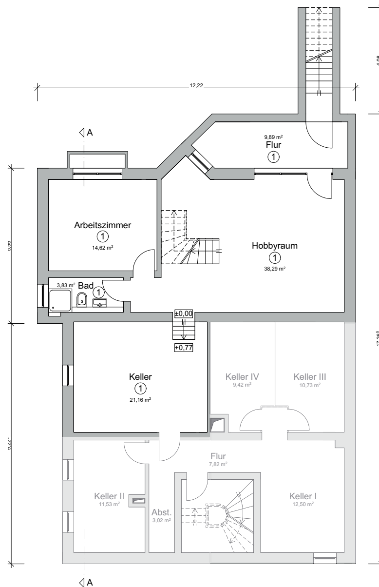
GRUNDRISS KELLERGEHOSS
