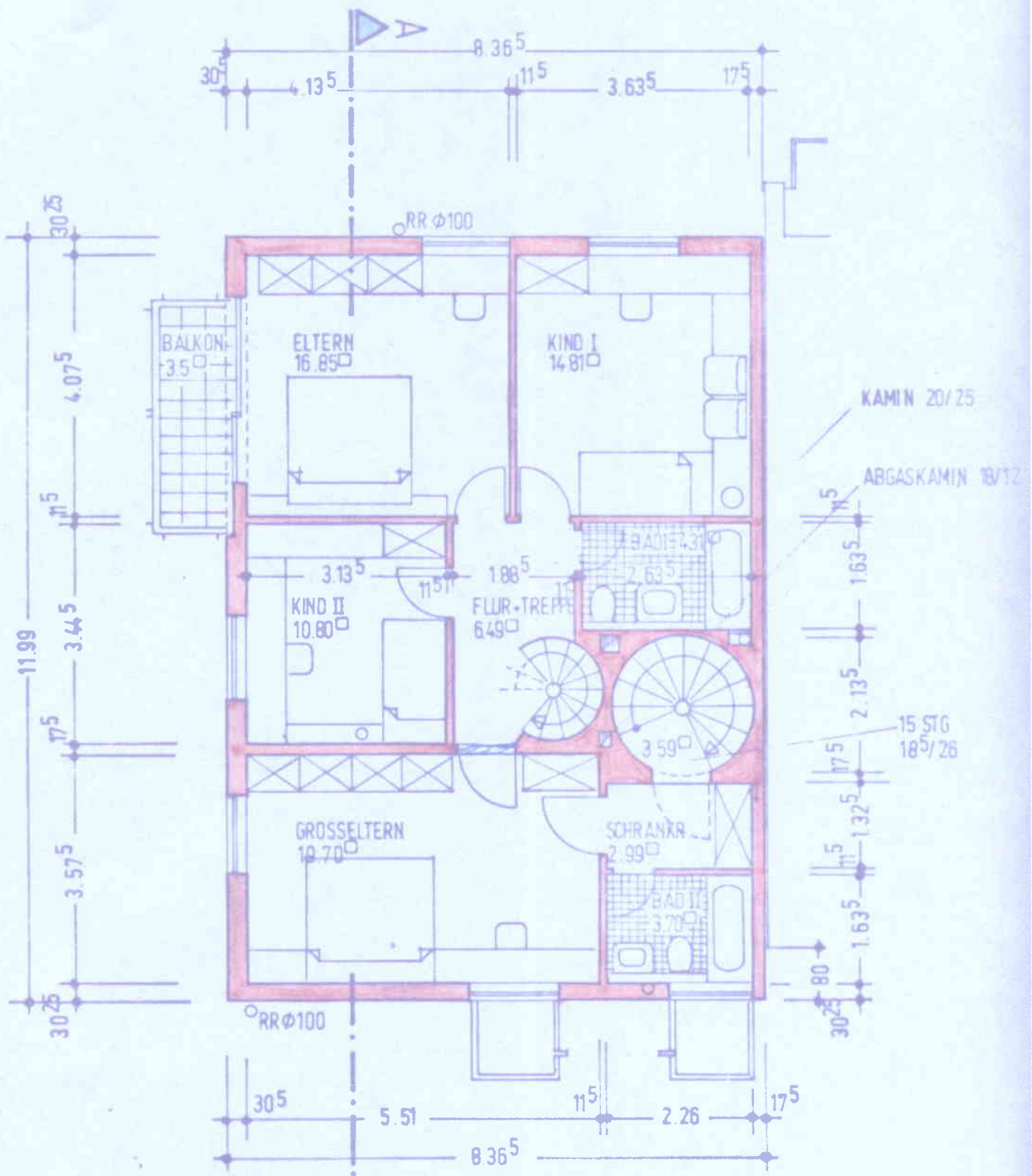
GRUNDRISS OBERGESCHOSS
