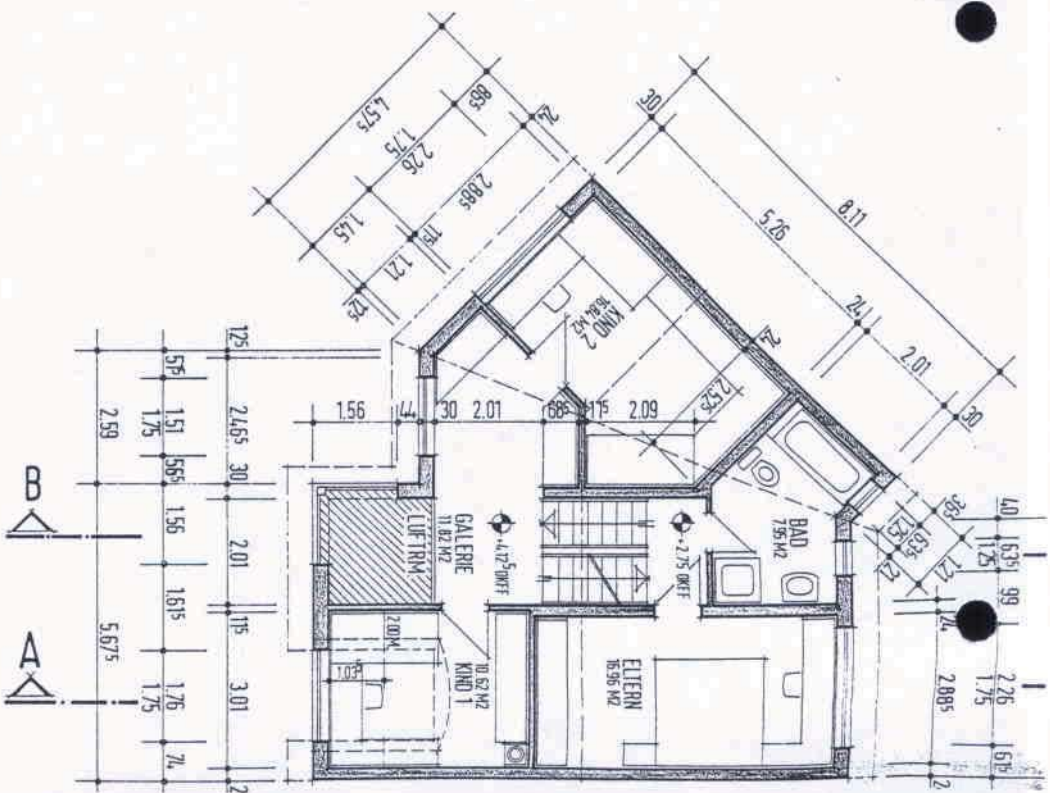
GRUNDRISS OBERGESCHOSS
