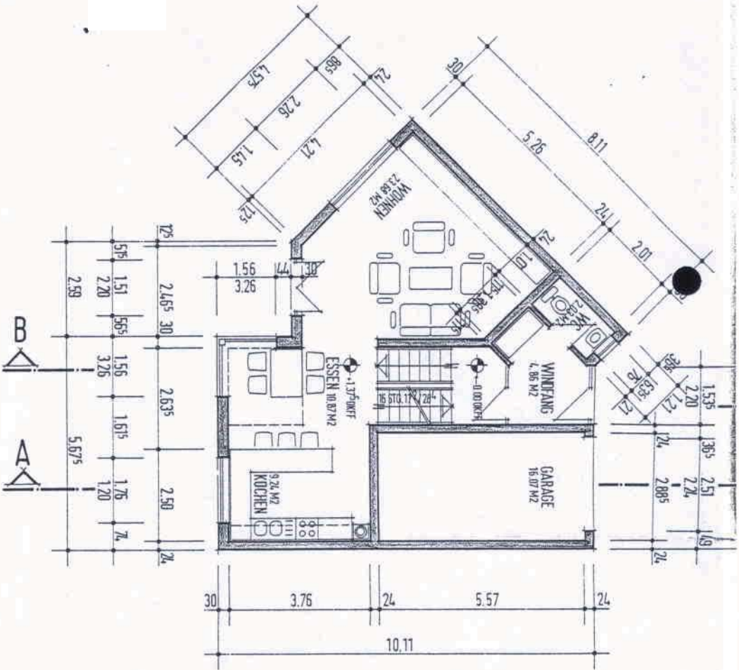
GRUNDRISS ERDGESCHOSS
